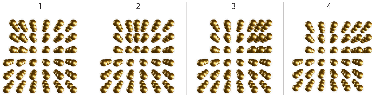
Ein wandernder Fehler: Eine Stufenversetzung, bei der eine Atomlage im Kristallgitter unvollständig ist, wandert durch einen Kristall, wenn ein Material verformt wird. In Bild 4 dieser schematischen Sequenz ist zu erkennen, wie sich daraus eine plastische Verformung ergibt.
