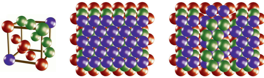
Falsch gestapelt: Die Farben der einzelnen Atomlagen stehen für die Positionen der Atome relativ zu den nächsten und übernächsten Atomlagen darunter. Die normale Anordnung für einen kubisch flächenzentrierten Kristall, dessen Elementarzelle links zu sehen ist, entspricht in dieser Darstellung der Abfolge Rot, Grün und Violett. Bei einem Stapelfehler sind die Positionen in einem Teilbereich verschoben (rechts), sodass sich die Stapelfolge Rot, Violett, Grün ergibt. Stapelfehler machen ein Material steifer; sie gezielt einzubauen macht einen Stahl fester.
