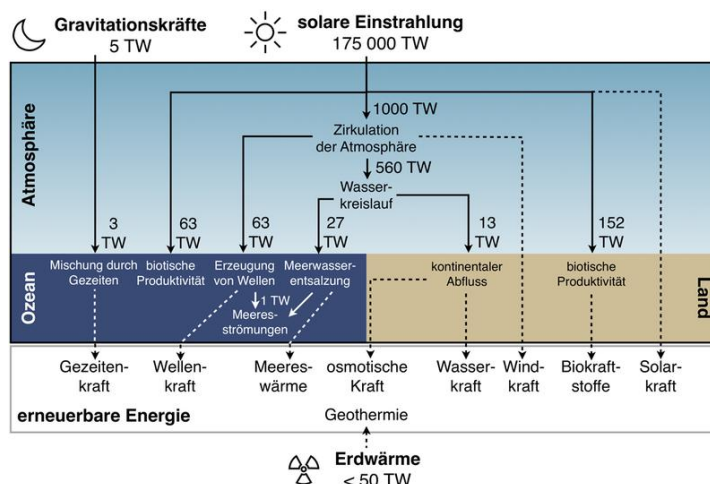
Abb. 2: Überblick von Energieumsatzraten im Erdsystem. Aus den drei Antrieben, solare Einstrahlung (175.000 TW = 175 \times 10^{15} W), Erdwärme (< 50 TW) und Gezeitenkräften (5 TW) erzeugen Erdsystemprozesse verschiedene Energieformen, die als erneuerbare Energien genutzt werden könnten. Zum Vergleich: Der globale Energieverbrauch der Menschheit im Jahr 2011 betrug 17 TW. Die Energieumsatzraten werden dargestellt in Einheiten der Leistung, also Arbeit pro Zeit, mit 1 \text{ TW} = 1 \text{ Terawatt} = 10^{12} \text{ W} . Nach [3, 5]. © Axel Kleidon, Max-Planck-Institut für Biogeochemie
