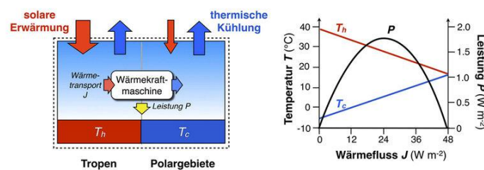
Abb. 1: Anwendung der Thermodynamik auf die maximale Leistung, die großskalige Windenergie erzeugen kann. Links: Unterschiede in solarer Einstrahlung zwischen Tropen und Polargebieten erzeugen Temperaturunterschiede (hier dargestellt durch die zwei Temperaturen, T_h (warm) und T_c (kalt)), die von der Atmosphäre in kinetische Energie umgesetzt werden können. Die dabei entstehenden Winde transportieren Wärme und verringern den Temperaturunterschied (rechts). Durch dieses Wechselspiel zwischen Wärmefluss und Temperaturunterschied gibt es eine Grenze der Leistung, die im Vergleich zur transportierten Wärme sehr gering ist. Nach [1-3].
